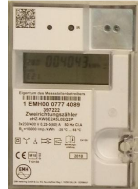
Stromzähler / Moderne Messeinrichtung
