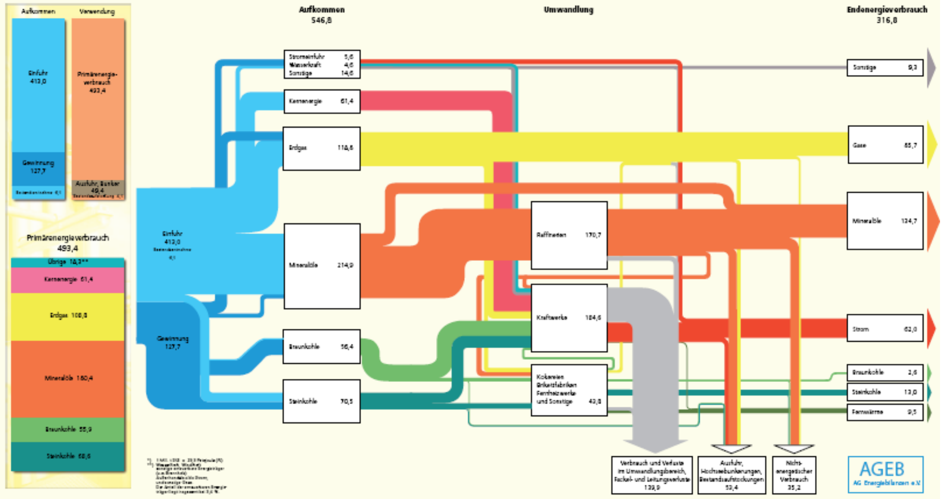
Energieflussbild der Bundesrepublik Deutschland 2003
